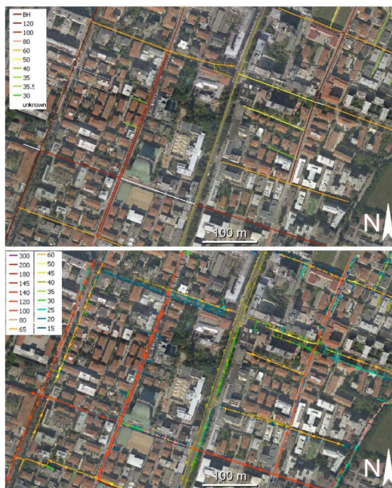
Figura 6. Confronto tra il livello conoscitivo pre (sopra) e post (sotto) ricognizione. I diversi colori rappresentano i diametri delle condotte.
