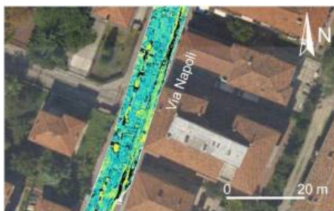
Figura 5. Esempio di sovrapposizione di time slice radar, calcolata al tempo di 20 ns, sul tratto mediano di Via Napoli.
