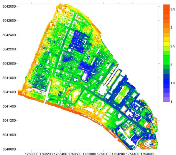
Figura 2. DTM del bacino fognario di Mestre – Via Torino.
