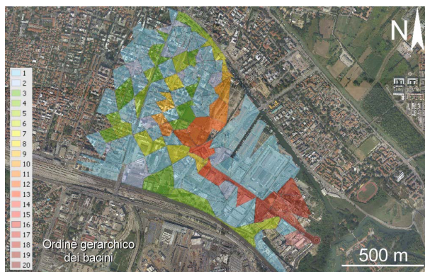
Figura 8. Schema dei sottobacini di raccolta delle acque meteoriche e reflue istituiti per il modello idraulico. Il colore rappresenta l'ordine gerarchico di ciascun bacino.
